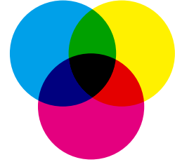
減法混合(色の三原色)
