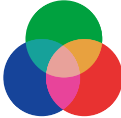
加法混合(光の三原色)
